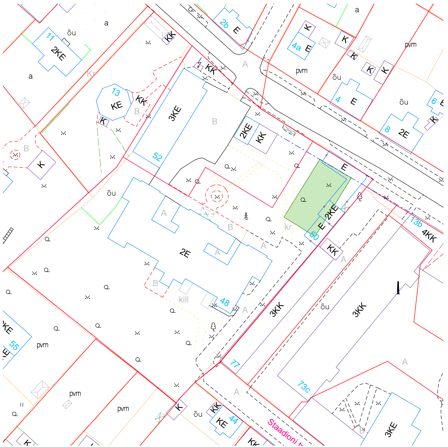
Lisa. Ehitusala skeem - Staadioni 81//83 PTH-20-021
